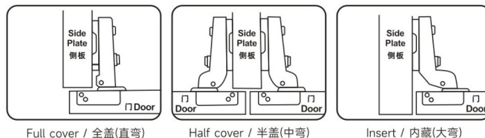
Full cover / 全盖(直弯)
